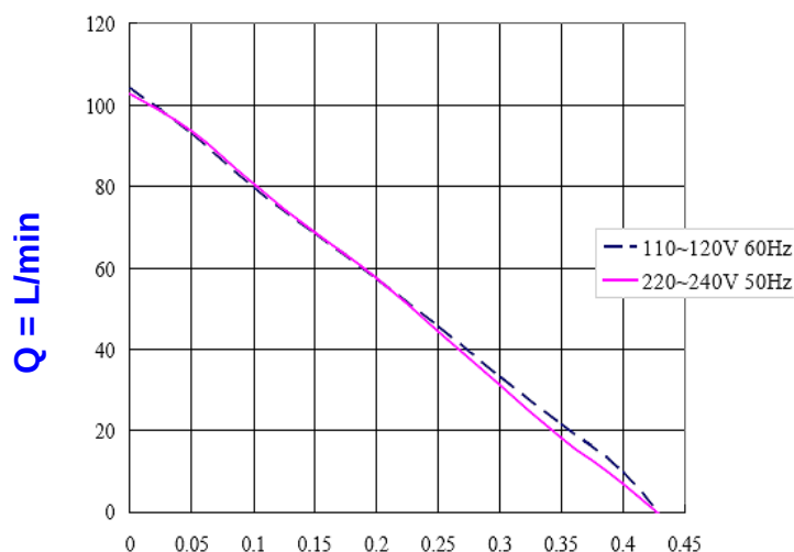
Výkonové křivky ( tolerance \pm 5\% )
